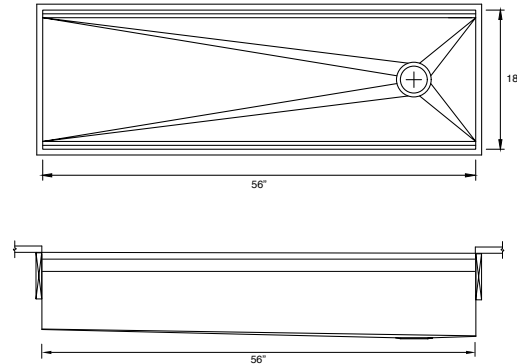
IWS-5-S-TT-xx
